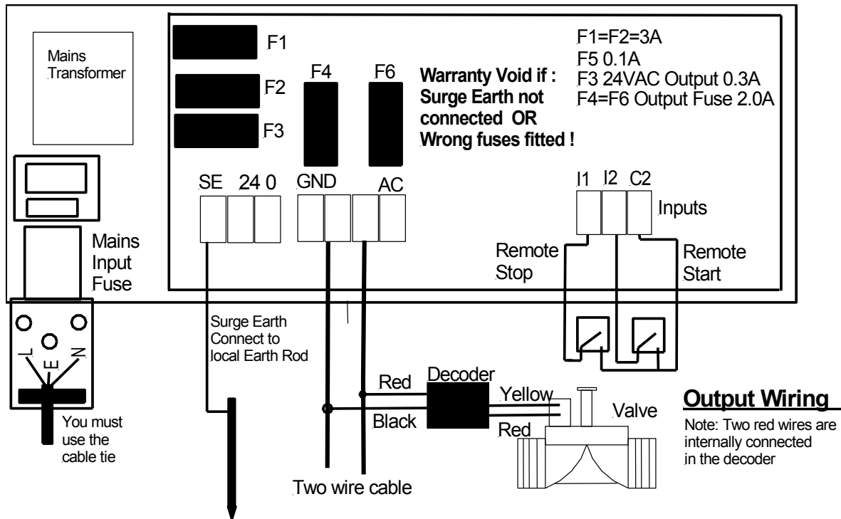
Fig 1 Output Wiring
